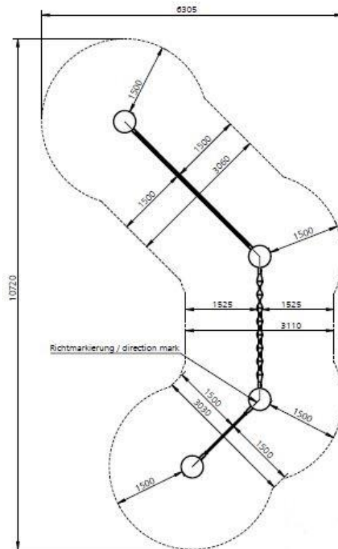
Wymiary strefy bezpieczeństwa
